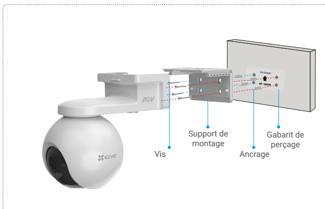
Fig. 2 Montage mural
